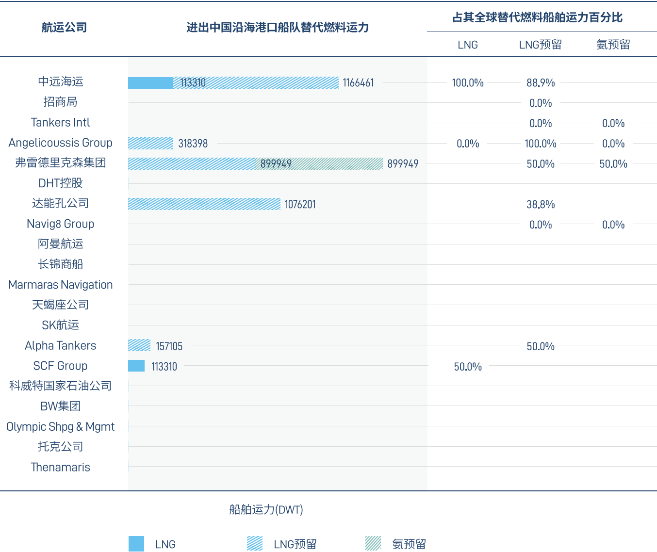
图 5.6 油轮航运公司参与中国国际海运的替代燃料船舶运力及占其全球替代燃料船舶的运力比重
