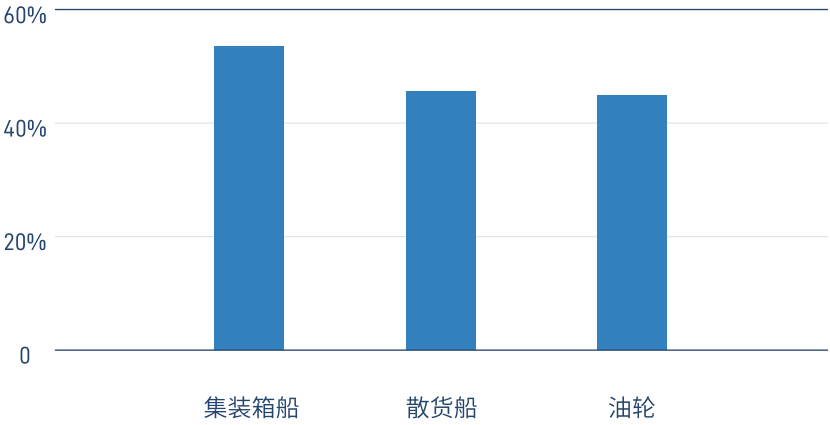
图 6.1 参与中国国际海运的船舶中 EEDI 生效后新造船的比例
