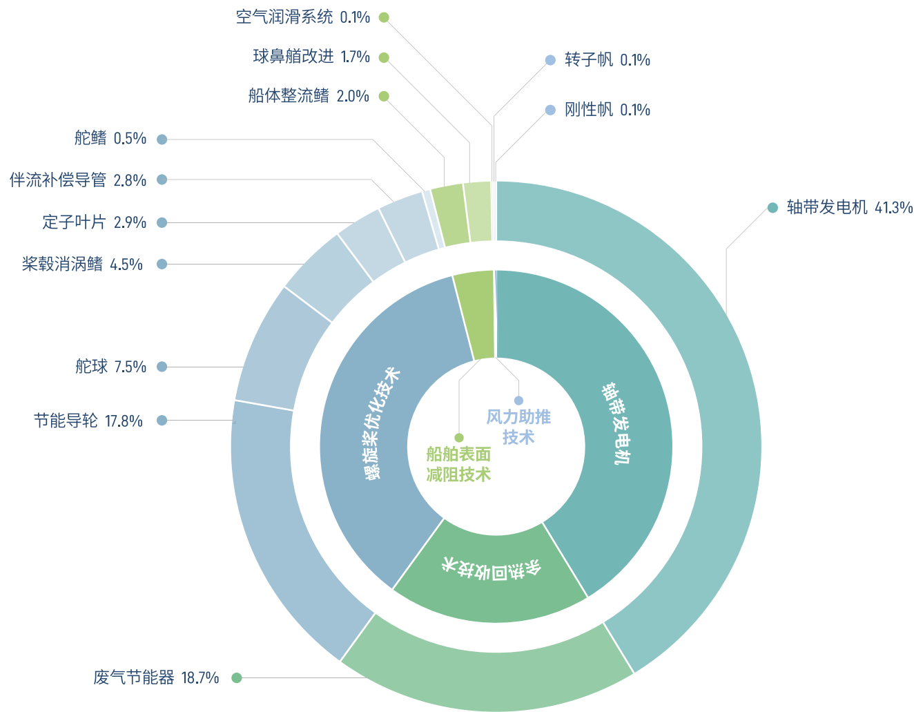
图4.6 油轮不同节能技术的应用比例
