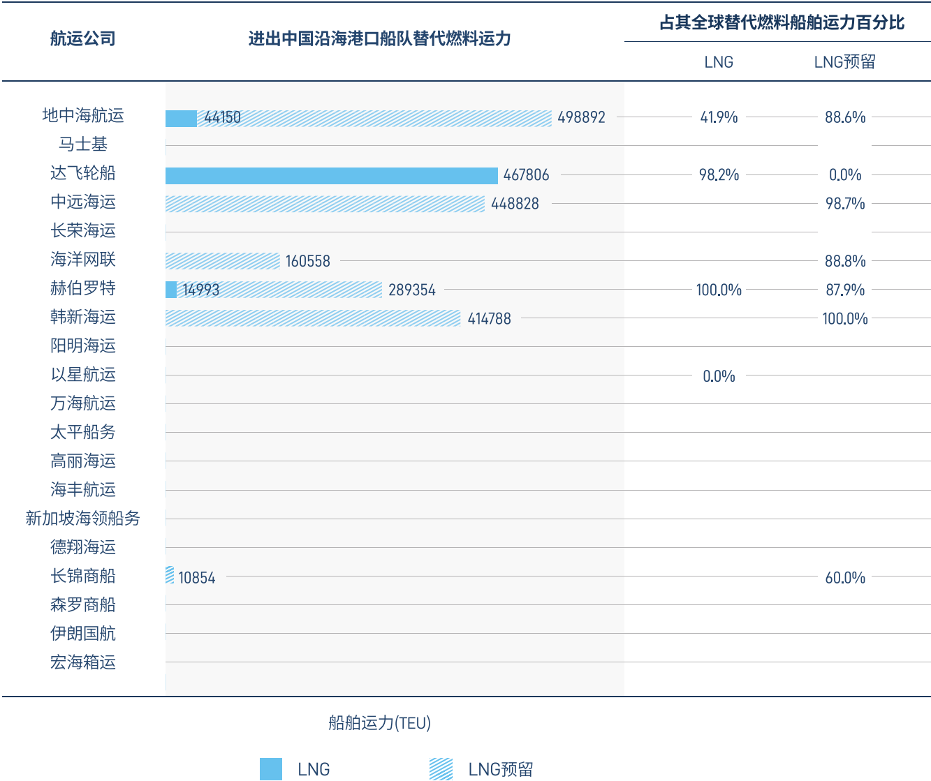
图 5.2 集装箱航运公司参与中国国际海运的替代燃料船舶运力及占其全球替代燃料船舶的运力比重
