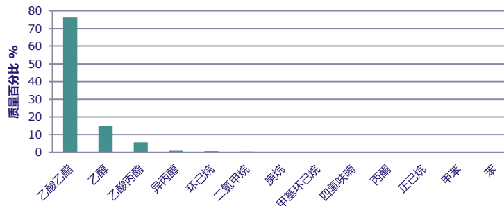
酯墨凹版印刷VOCs组分构成
