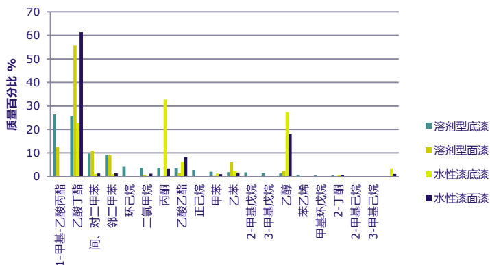
木质家具制造业VOCs组分构成
