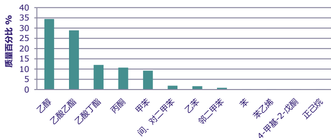
电缆行业VOCs组分构成
