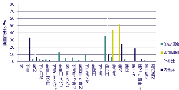
制罐行业VOCs组分构成
