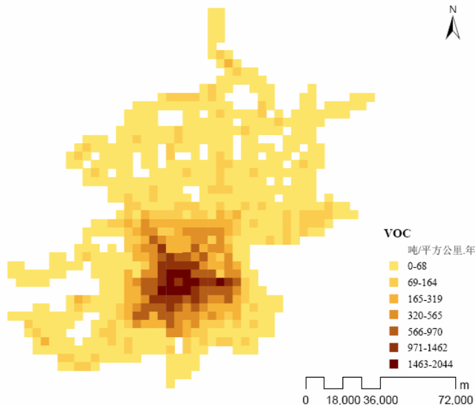
北京机动车VOCs排放空间分布
