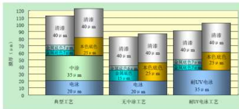
机动车制造企业采用 无中涂涂装工艺
